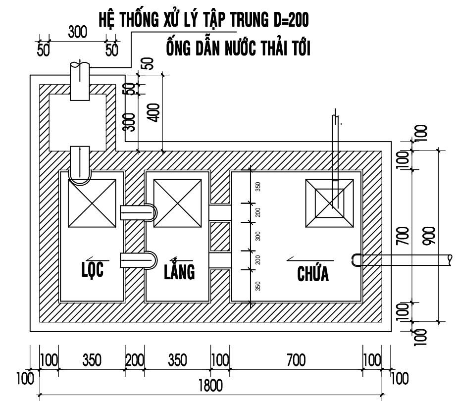
MẶT CẮT BỂ TỰ HOẠI
