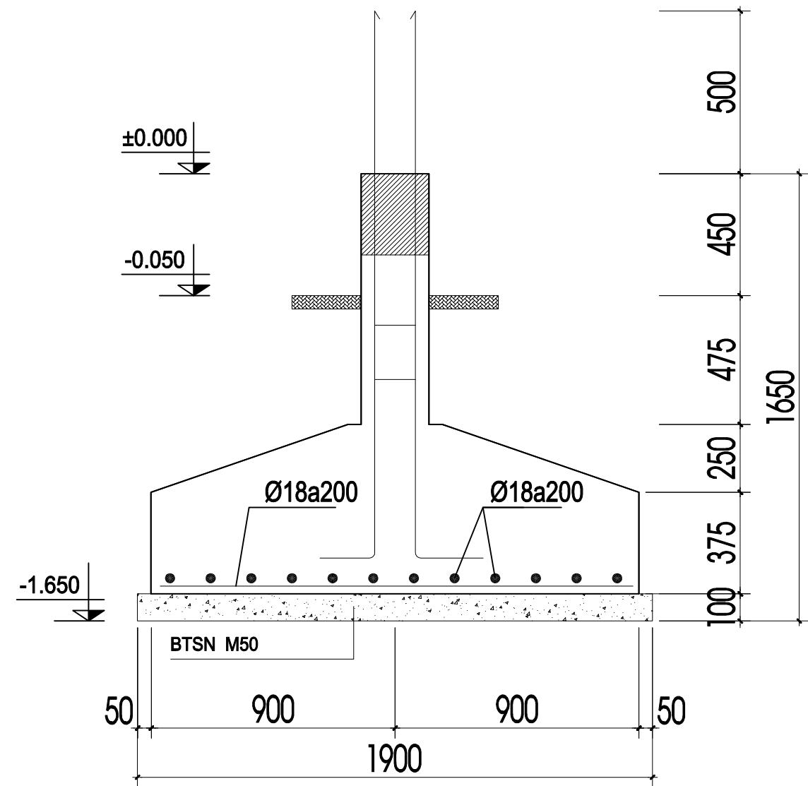
CHI TIẾT MÓNG M-2
