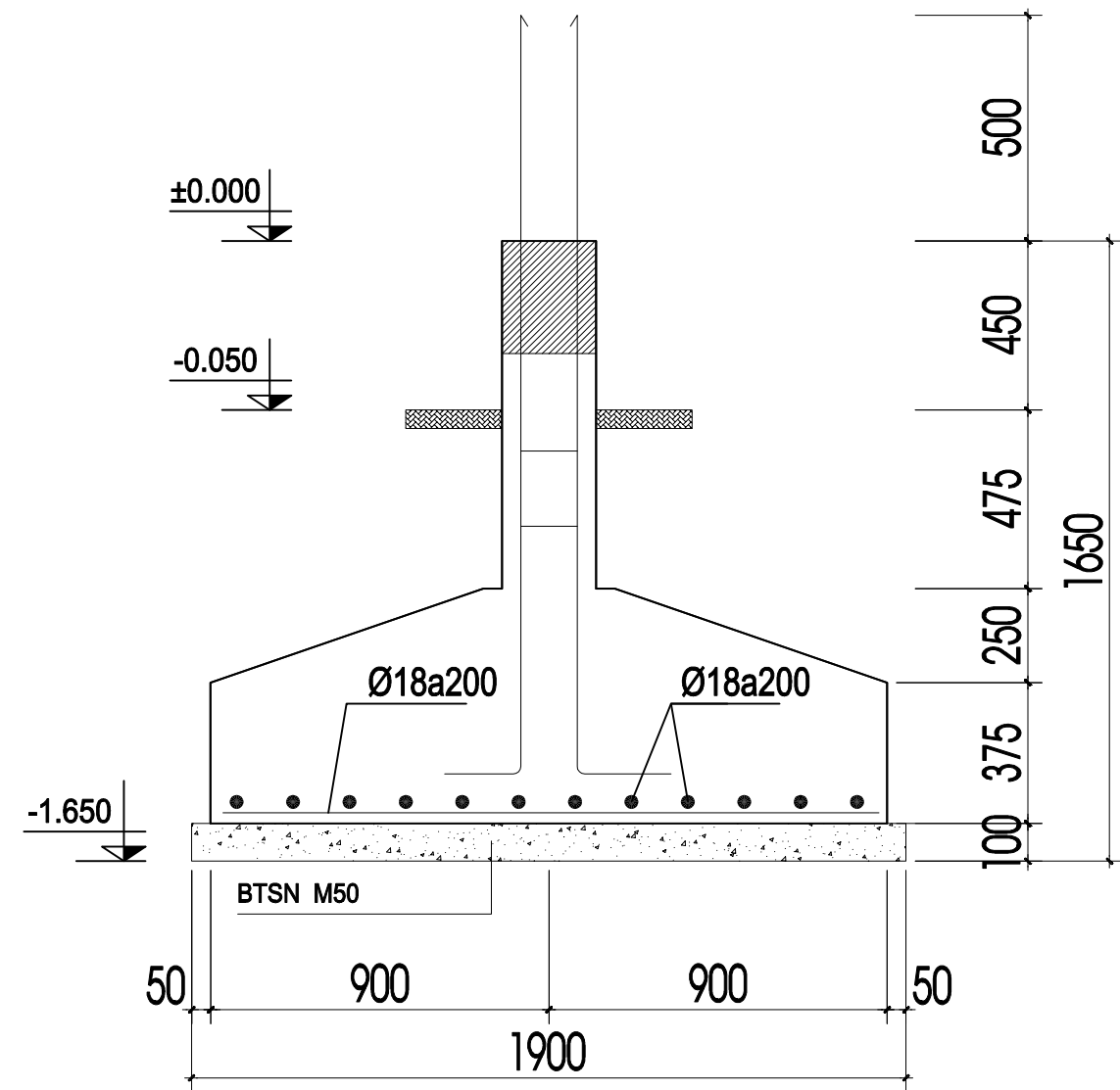
CHI TIẾT MÓNG M-3
